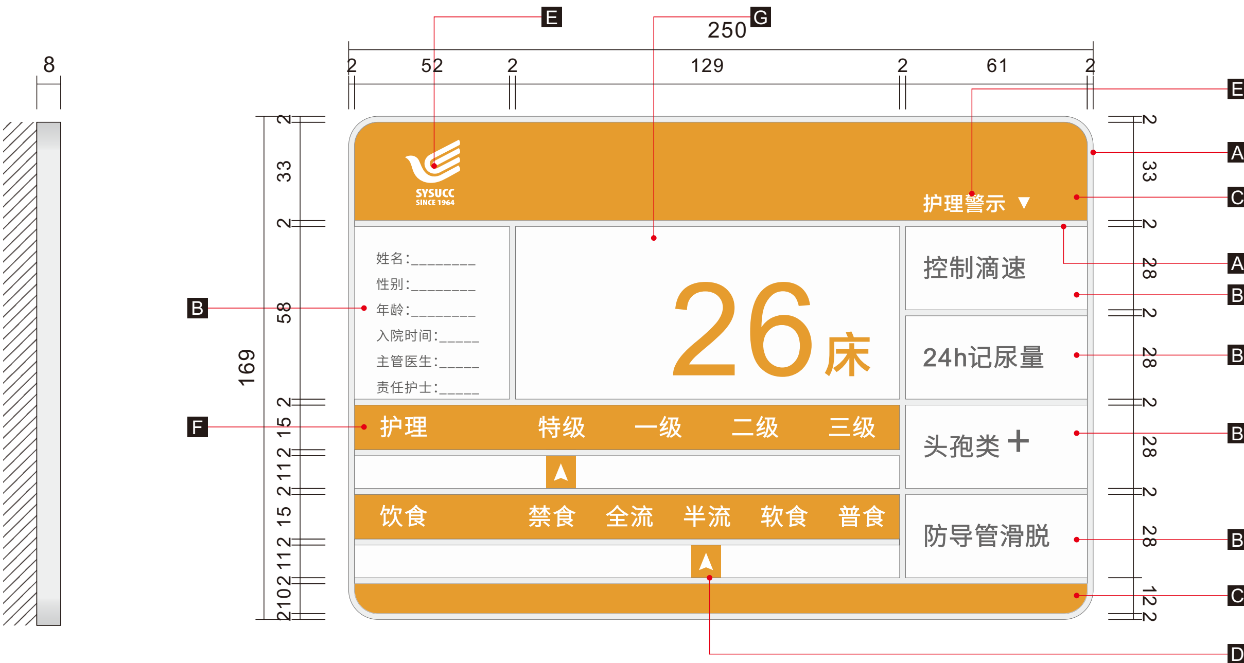
左视图 LEFT VIEW
