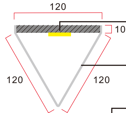
俯视图剖面图
