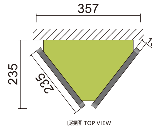
顶视图 TOP VIEW
