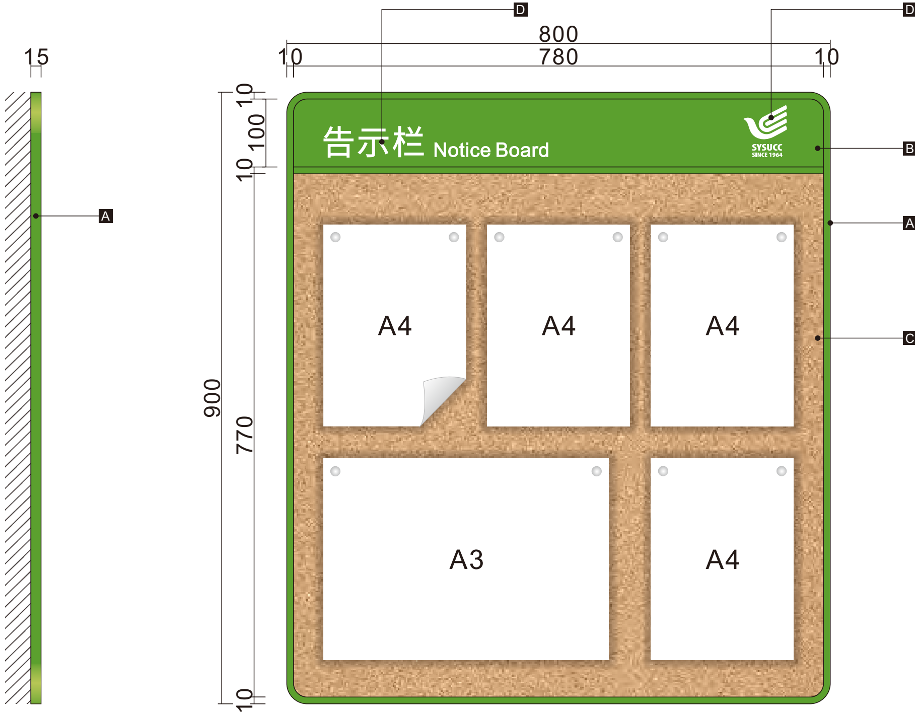
左视图 LEFT VIEW
