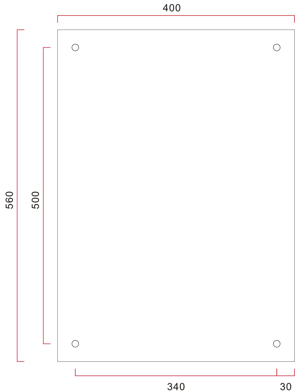
正视图
